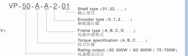
Motor / 馬達
