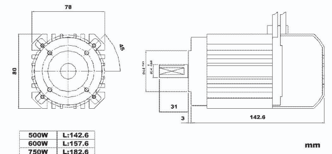
Motor / 馬達
